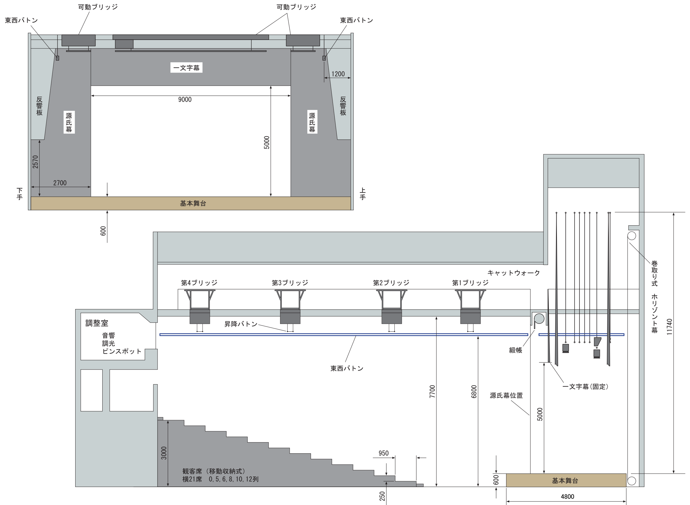
名称 タウンホール基本舞立面図/正面図 縮尺 1/100
